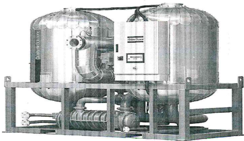
Конструктивное исполнение адсорбционного осушителя с регенерацией адсорбента теплом компримирования
