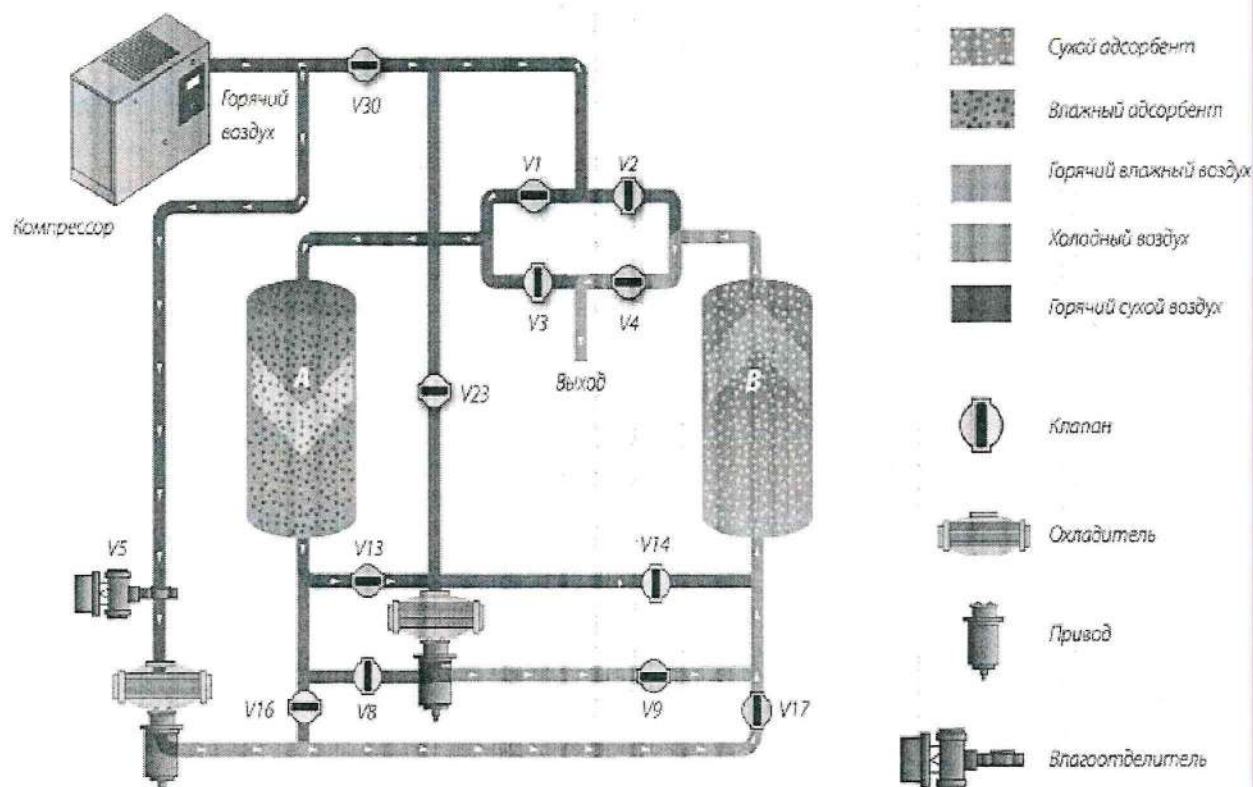
Принципиальная схема адсорбционного осушителя с регенерацией адсорбента теплом компримирования
